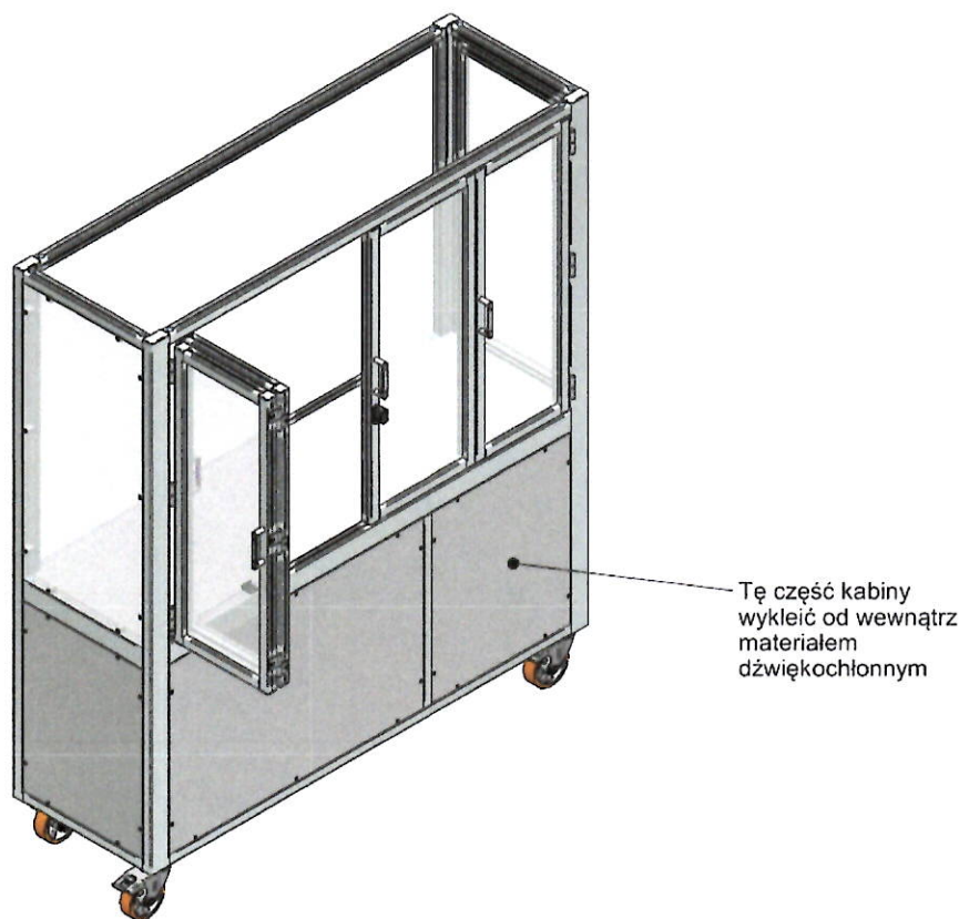
Rys. 1 Schemat ogólny obudowy stanowiska
